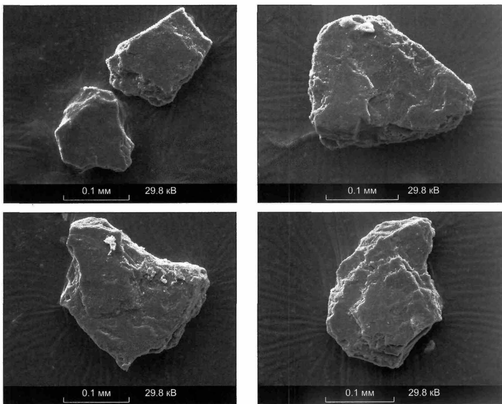
Рис. 4. Фотографии зерен хлоритоида из позднелейстоценовых отложений (колонка 04-2), сделанные на электронном сканирующем микроскопе PHILIPS M525 в ЦПК «Электронная микроскопия» при ЛИН СО РАН.
