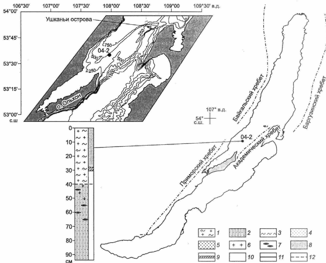
Рис. 1. Схема оз. Байкал с точкой отбора керна и литологическое строение разреза 04-2 (Академический хребет).
