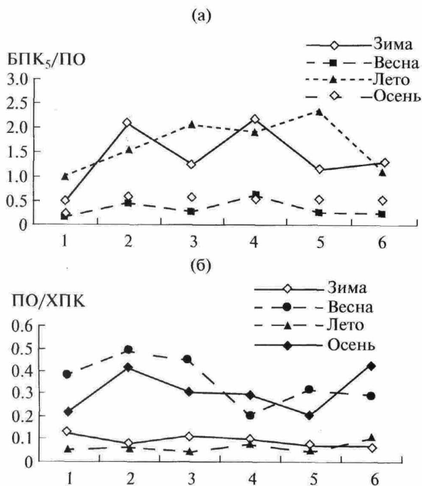
Рис. 3. Внутригодовое и пространственное изменение соотношений БПК 5 /ПО (а) и ПО/ХПК (б) в воде р. Селенги. 1 – пос. Наушки, 2 – с. Новоселенгинск, 3 – выше г. Улан-Удэ, 4 – ниже г. Улан-Удэ, 5 – ниже с. Тресково, 6 – пос. Кабанск.
